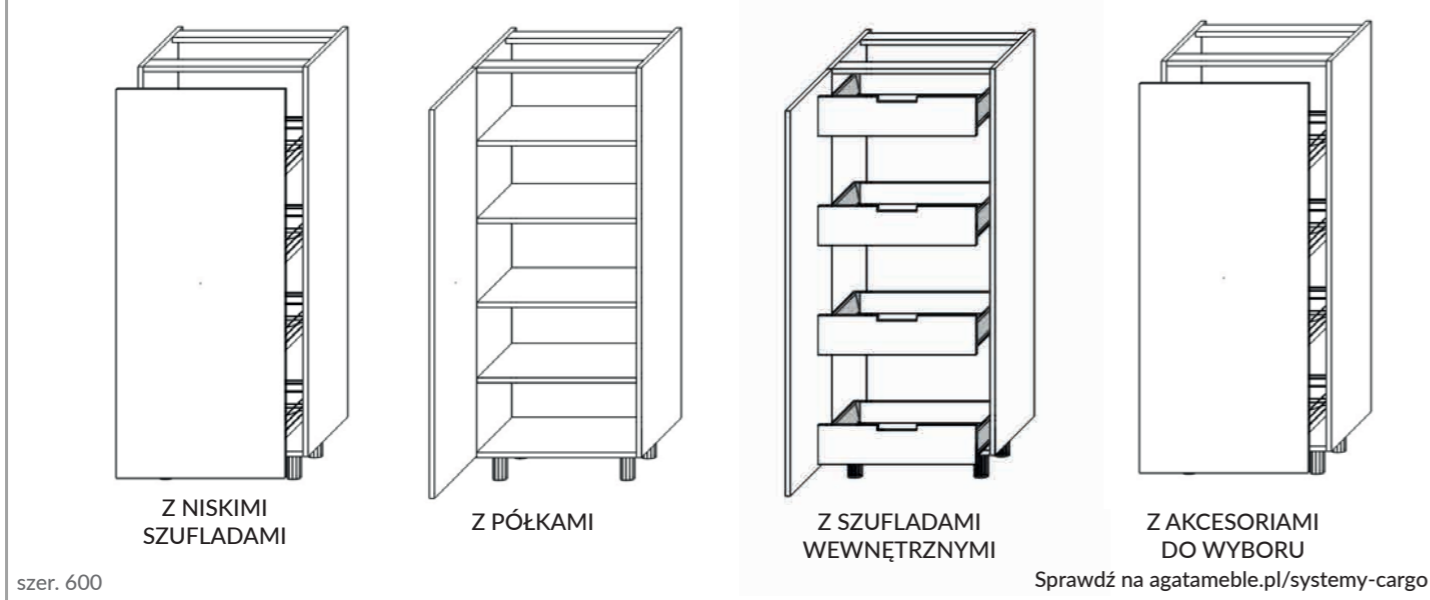
wys. 1478 SZAFKI DOLNE Z CARGO
