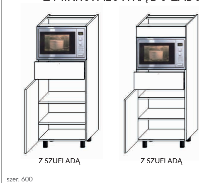
wys. 1478 Z MIKROFALÓWKĄ DO ZABUDOWY
