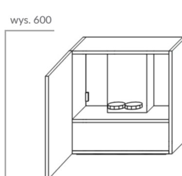
SZAFKA Z OKAPEM ERA C IX/A/52
